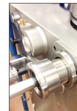
Füllrohrträger Handwerk Sortenwechsel mit minimalen Brätresten Stuffing horn support for small trade business Product changeover with minimal residues
