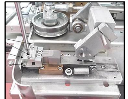
Prägeeinheit zur Kennzeichnung
